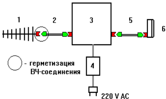
Схема соединений
